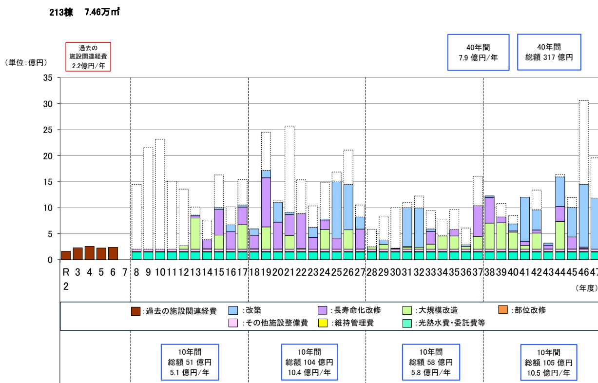
◆図表 8-4 今後の維持・更新コスト（中・長期計画）
